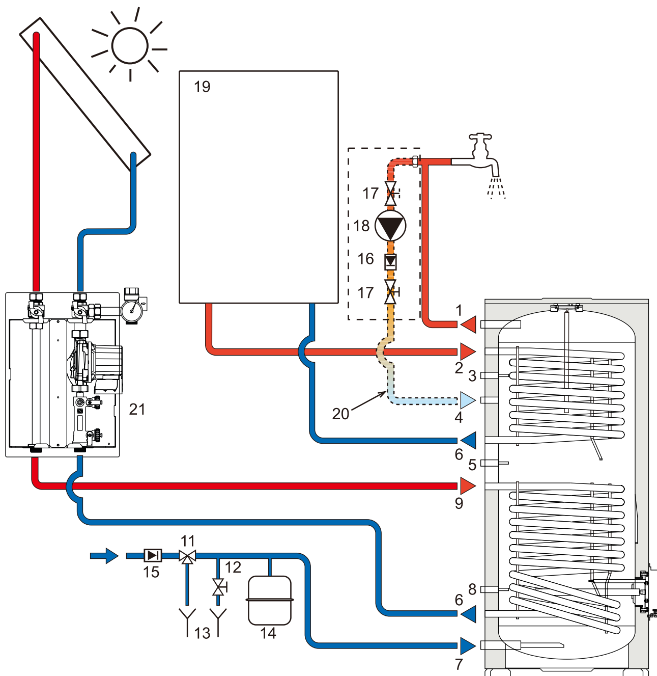
Рис. 6 – Гидравлический контур ECOUNTIT N 2C
