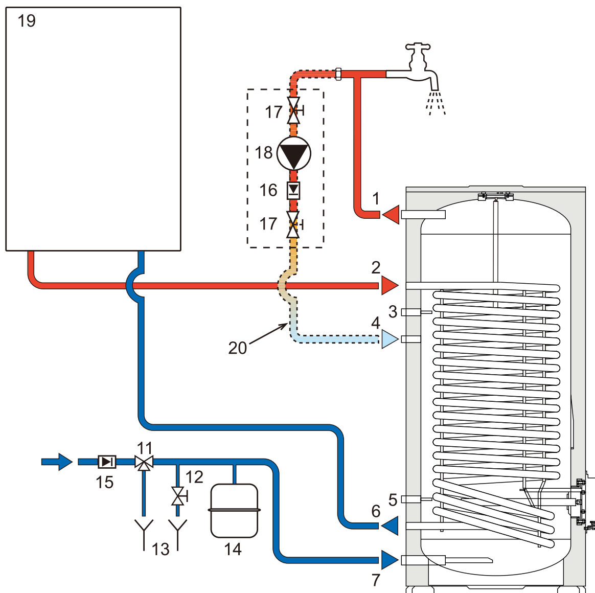
Рис. 5 – Гидравлический контур ECOUNTIT N 1C
