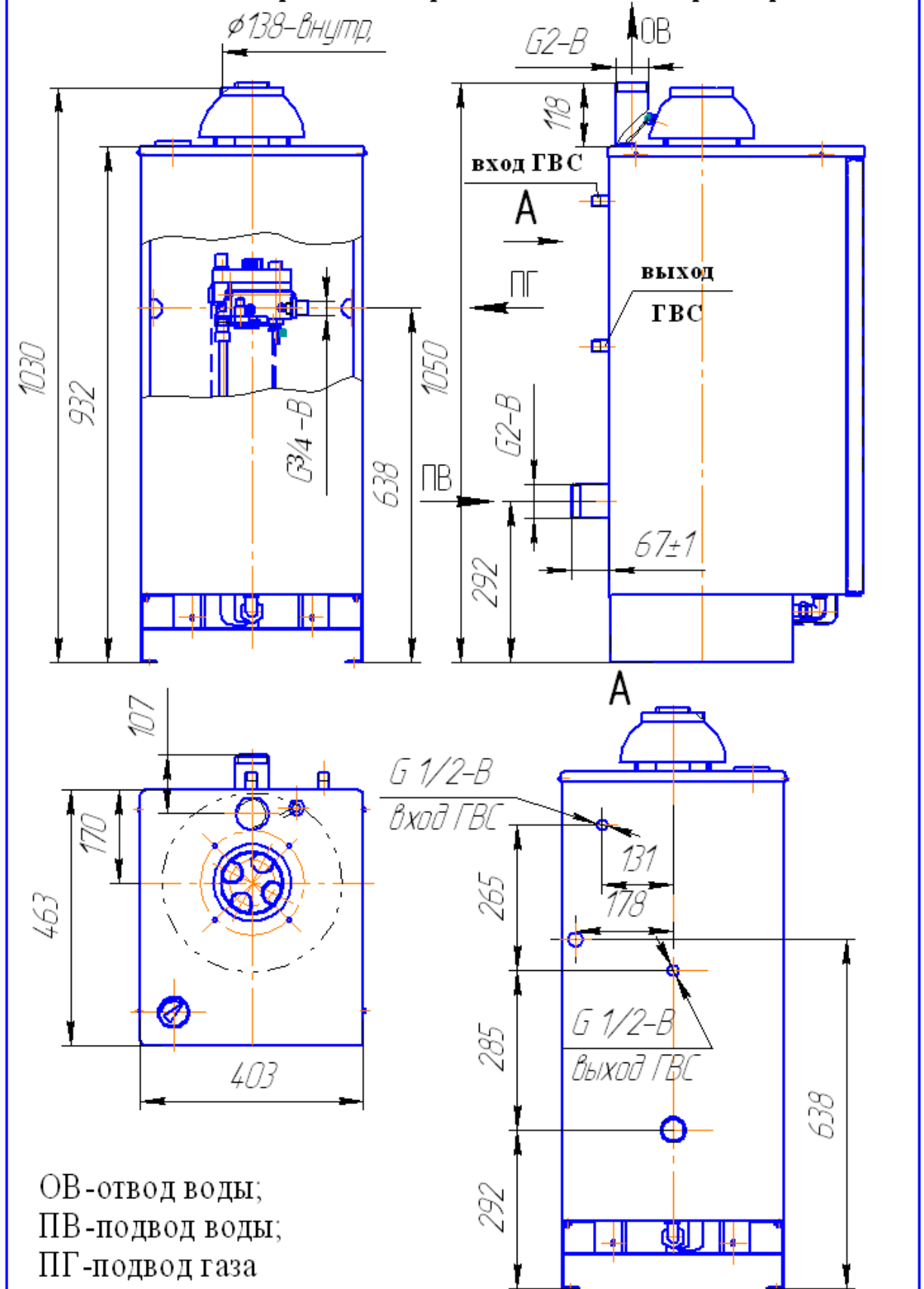
Рис.2 Габаритные и присоединительные размеры
