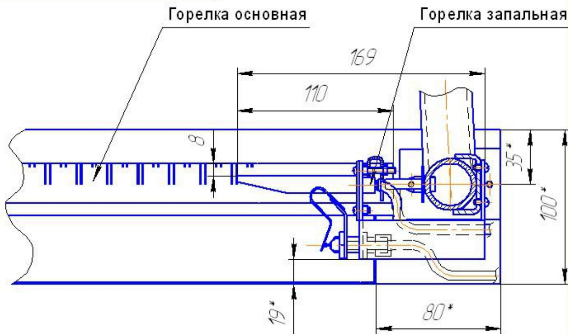
Рис.2А Схема расположения запальной горелки относительно основной.
